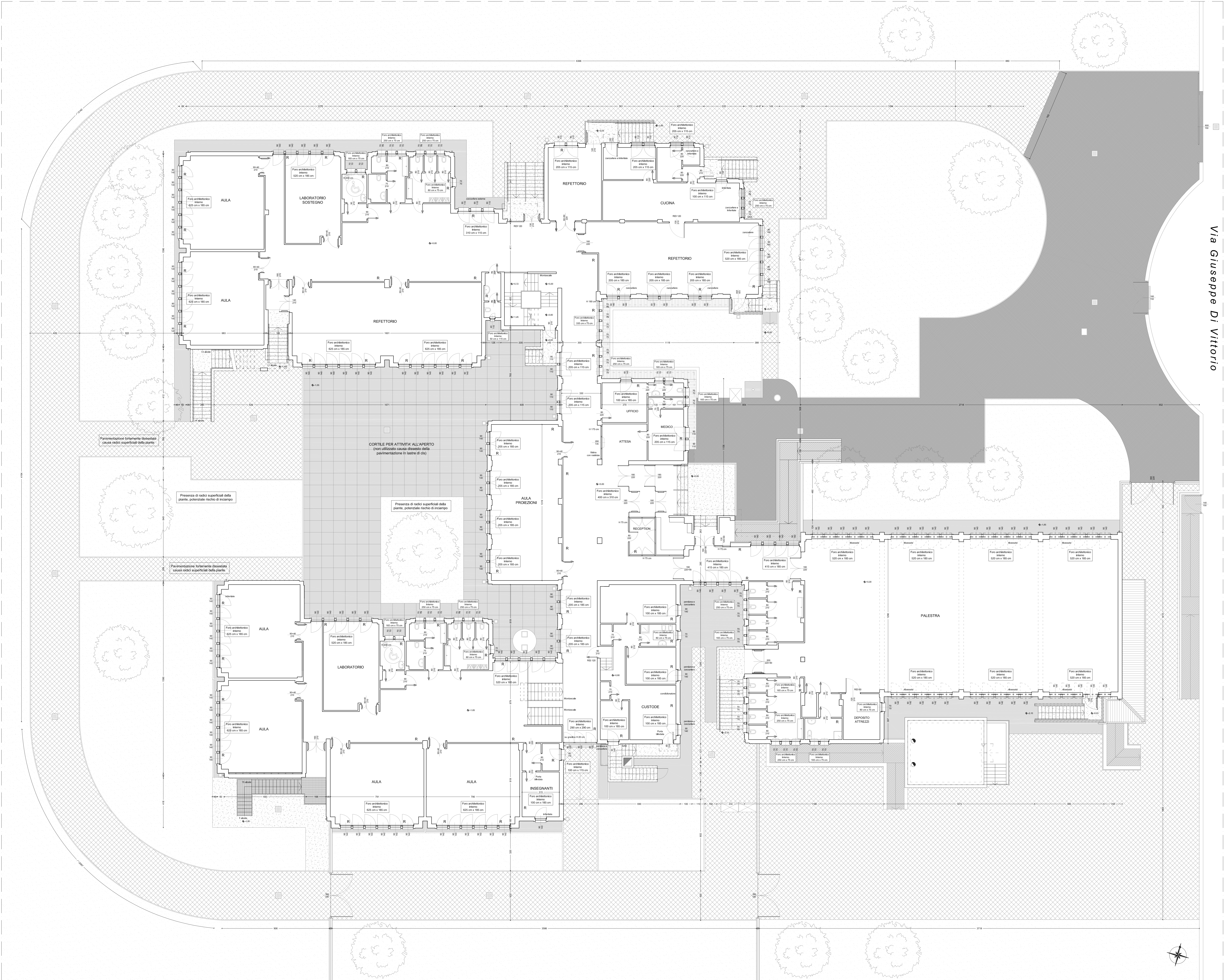
PLANIMETRIA GENERALE DELLA SCUOLA - PIANO RIALZATO +0.00 m / +1.65 m
