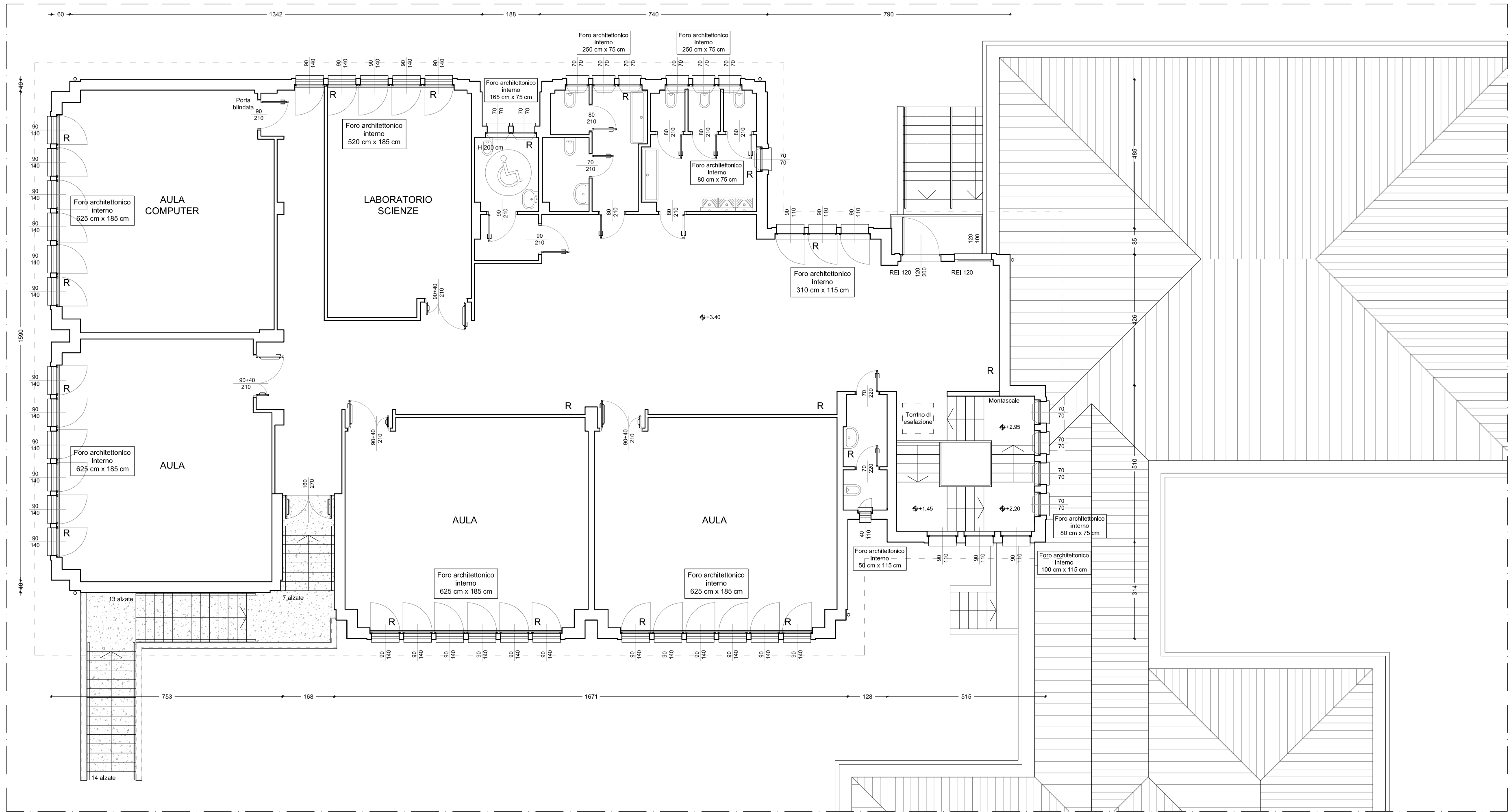
PLANIMETRIA PIANO PRIMO +3.40 m
