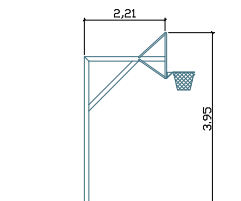
VISTA LATERALE
