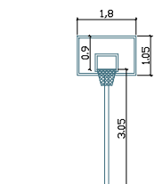
VISTA FRONTALE
